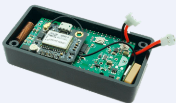
LoRa GPS-tracker met open hard- en software
